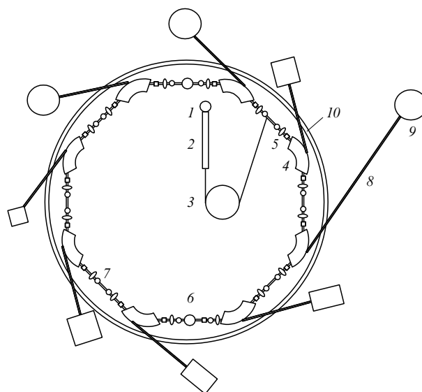
Рис. 3. Общее устройство накопительного кольца — источника СИ. 1 — электронная пушка, 2 — линейный предускоритель (лиак), 3 — кольцевой предускоритель (бустер), 4 — поворотный магнит, 5 — система магнитных линз, 6 — радиочастотный резонатор, 7 — линейный участок камеры для размещения специализированных магнитных (встроенных) устройств, 8 — канал, 9 — экспериментальная станция, 10 — бетонная стена биозащиты.
