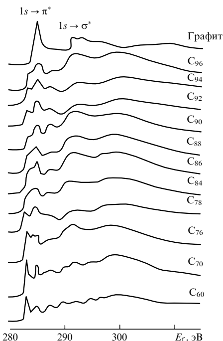
Рис. 11. Спектры NEXAFS на K -крае атома углерода для ряда фуллеренов C_n ( n = 60–96 ). Указаны электронные переходы, вносящие основной вклад в соответствующие спектры поглощения. 58
