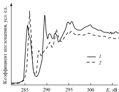
Рис. 29. Микрондвовые спектры NEXAFS ( K -край C), полученные для тонких полимерных пленок площадью 0.1 мкм 2 с помощью сканирующего рентгеновского микроскопа (синхротронный центр NSLS). 212
