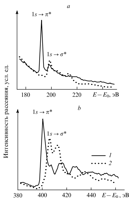
Рис. 22. Тонкая структура К-краев поглощения бора (a) и азота (b) по данным рентгеновского рамановского рассеяния на монокристалле нитрида бора в режиме пропускания (1) и отражения (2). 180 1 — вектор рассеяния параллелен оси c , 2 — вектор рассеяния перпендикулярен оси c ; возбуждающая энергия \sim 7 кэВ.
