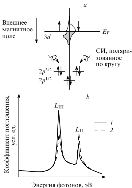
Рис. 25. Схема, иллюстрирующая возникновение кругового дихроизма в спектрах рентгеновского поглощения (а), и типичный спектр кругового дихроизма на L_{II} , III -краях 3d - и 4d -металлов (б). Поляризация возбуждающего излучения выбрана так, что спин возбуждаемого электрона параллелен (1) и антипараллелен (2) направлению внешнего магнитного поля.
