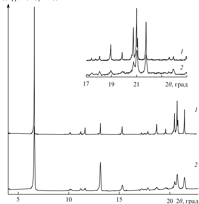
Рис. 18. Порошковые дифрактограммы образца ион-радикальной соли \text{BEDTTTF}^+ \cdot \text{C}_{60} \cdot \text{I}_3^- (BEDTTTF — бисэтилендитиотетратиафульвален).
