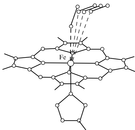
Рис. 31. Миграция CO (штриховые линии) на начальных стадиях декарбонилирования комплекса миоглобина с CO, инициируемого вспышкой видимого света (синхротронный центр ESRF). Положения получены уточнением исходной структурной модели по серии лауэграмм для монокристалла миоглобина с разрешением во времени \sim 10 пс. 392
