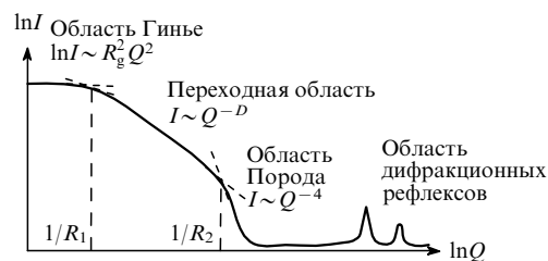
Рис. 20. Общий вид кривой малоуглового рассеяния на неоднородном объекте.
