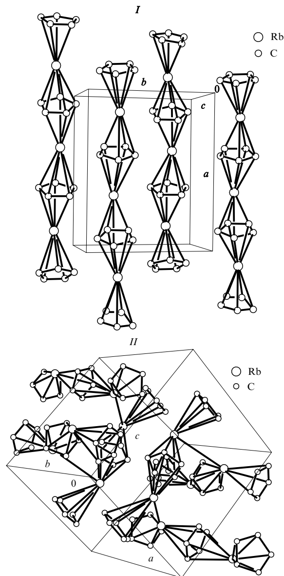
Рис. 19. Кристаллические структуры полиморфных модификаций \text{Rb}(\text{C}_5\text{H}_5) , различающиеся мотивом упаковки бесконечных цепочек \text{C}_5\text{H}_5 - \text{Rb} - \text{C}_5\text{H}_5 . Структуры расшифрованы ab initio по порошковой дифрактограмме их смеси. 154
