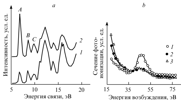
Рис. 14. Фотоэлектронные спектры валентной зоны \pi -комплекса \text{Ti}(\eta^7\text{-C}_7\text{H}_7)(\eta^5\text{-C}_5\text{H}_5) при различных энергиях возбуждения (а) и зависимость относительных сечений фотоионизации для полос А, В, С от энергии возбуждения (б). 77 а: энергия возбуждения, эВ: 1 — 33, 2 — 48; б: полоса: 1 — А, 2 — В, 3 — С. Резкое увеличение интенсивности полосы А в области ~48 эВ, связанное с приближением возбуждающей энергии к M_{II,III} -краю поглощения Ti ( 3p \rightarrow 3d -резонанс), указывает, что в соответствующую молекулярную орбиталь основной вклад вносит 3d -атомная орбиталь титана; полосам В и С соответствуют молекулярные орбитали со значительным вкладом орбиталей лигандов.
