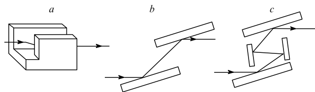
Рис. 7. Примеры рентгеновских монохроматоров.
