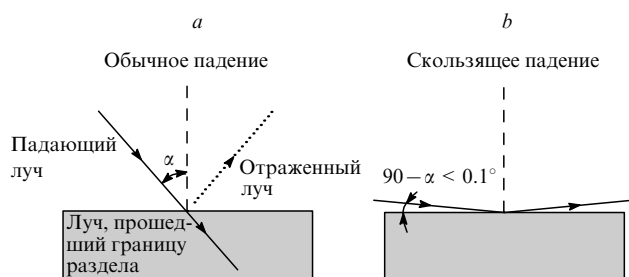
Рис. 9. Отражение рентгеновского пучка от поверхности в условиях обычного (a) и скользящего (b) падения.
