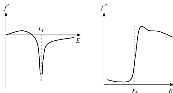
Рис. 24. Зависимость действительной ( f' ) и мнимой ( f'' ) частей аномально-дисперсионной поправки к атомному фактору рентгеновского рассеяния от энергии рассеиваемого излучения.
