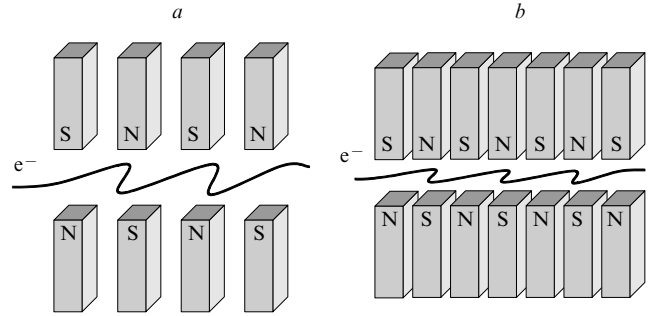
Рис. 4. Специализированные магнитные устройства — виглер (a) и ондулятор (b).
